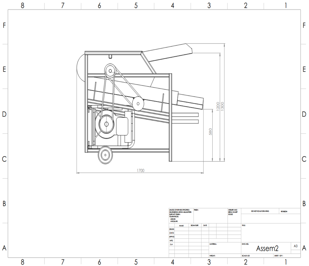
Hình 2: Bản thiết kế thiết bị tước quả
